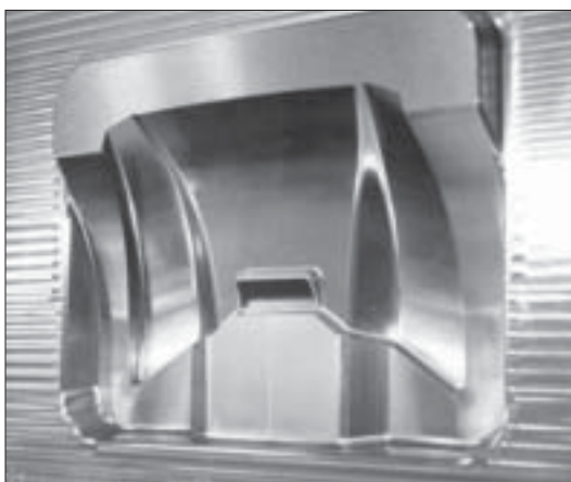
Forstærkningsdel for rygstøtte til stol
